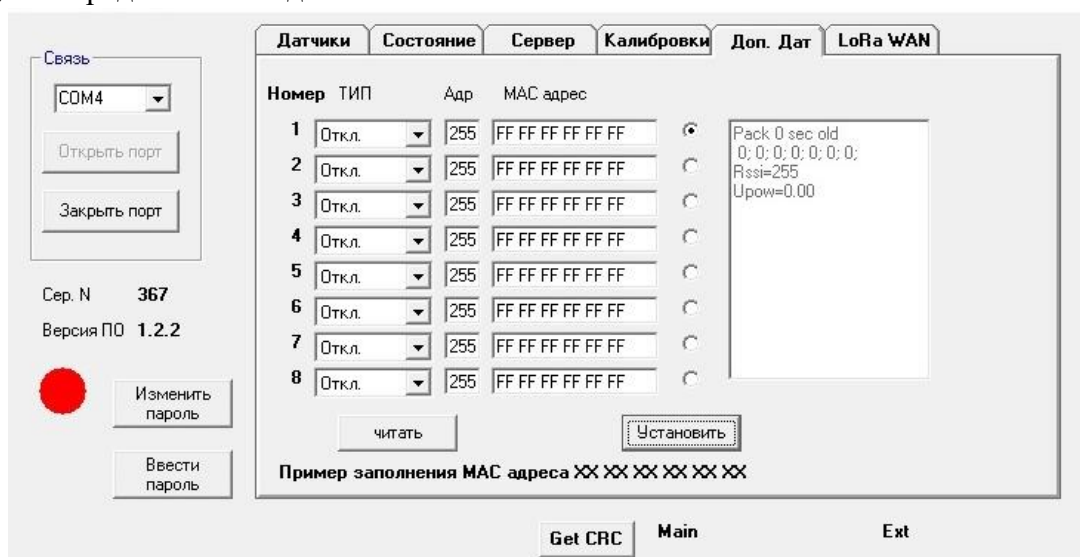
Рисунок 7 – «SokolCFG» вкладка «Доп.Дат»
