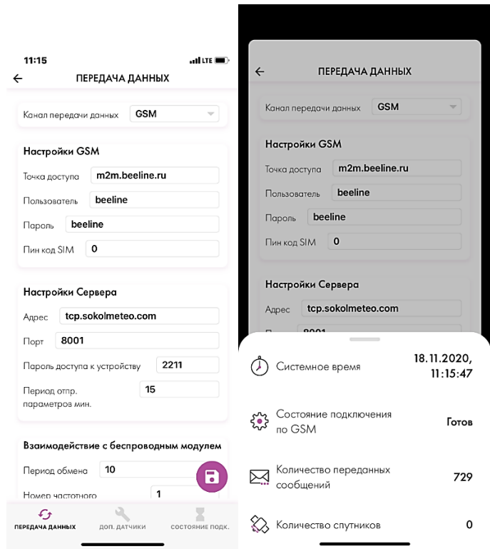
Рисунок 33 – Окно Конфигуратора
