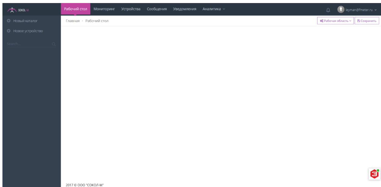
Рисунок 13 – Главная страница
