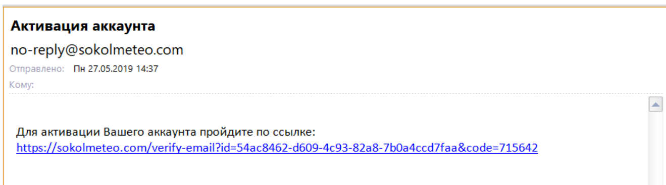
Рисунок 11 – Активация аккаунта
