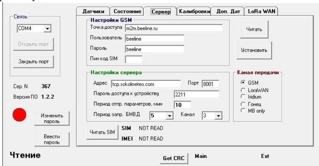
Рисунок 6 – «SokolCFG» вкладка «Сервер»
