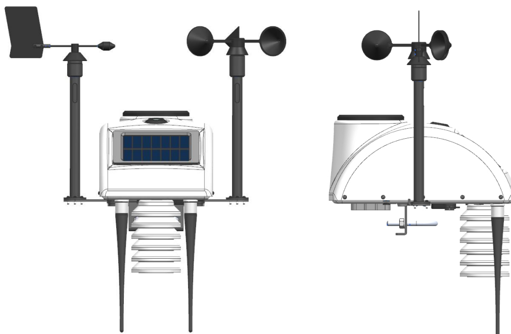
Рисунок 1 – Внешний вид метеостанции СОКОЛ-М1
